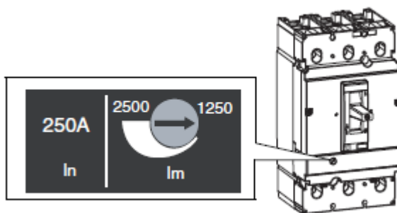
Figure 6 - PowerPacT J FLA and Im Dial
