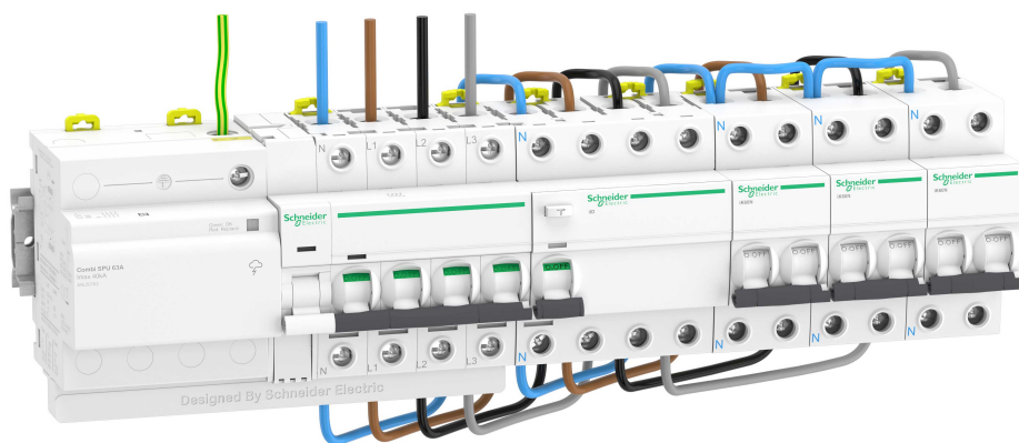
Figura 2: configuración típica del cableado de una instalación de Combi SPU 3P + N
