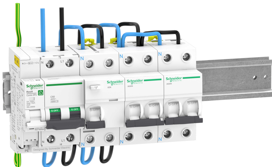
Figura 1: configuración típica del cableado de una instalación de Combi SPU 1P + N
