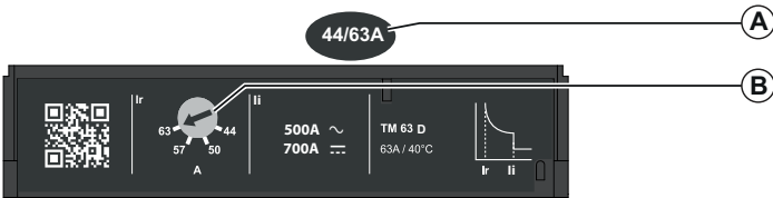
A TM-D 热磁 3P/4P 脱扣单元的设置范围 B 用于热保护吸合电流 I_r 的调节旋钮
