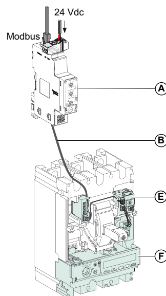
示例 4：将 IFM 通讯接口连接到 BSCM Modbus SL/ULP 模块及 MicroLogic 5、6 或 7 脱扣单元
