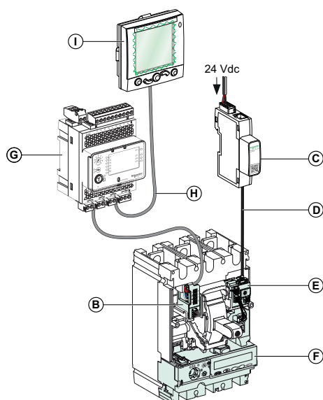
示例 3：将 IFM 通讯接口连接到 BSCM Modbus SL/ULP 模块
