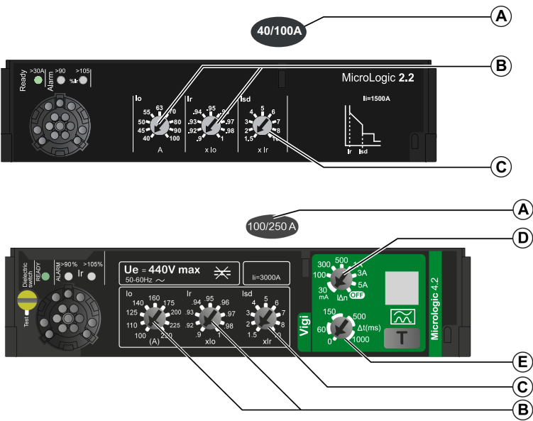
示例 22：MicroLogic 和 MicroLogic 4 电子脱扣单元
