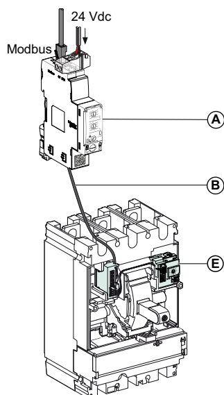
示例 3：将 IFM 通讯接口连接到 BSCM Modbus SL/ULP 模块
