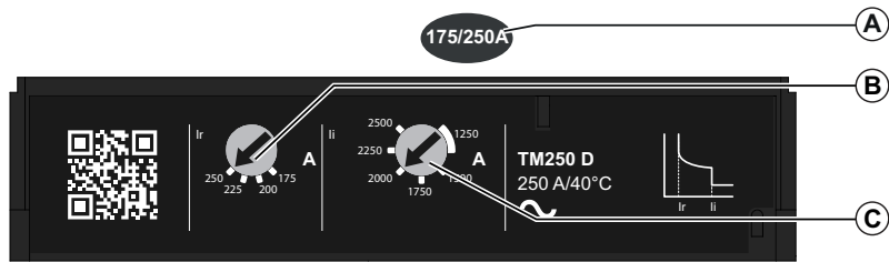
示例 1：TM-D 热磁脱扣单元
