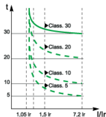
标准脱扣时间值
