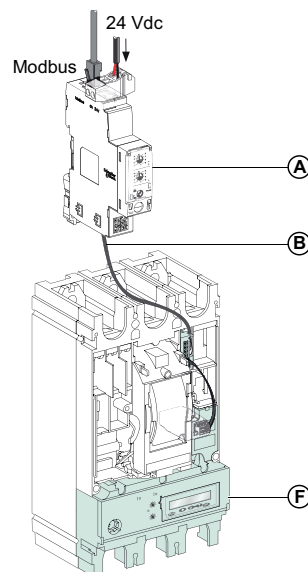
示例 2：将 IFM 通讯接口连接到 MicroLogic 5、6 或 7 脱扣单元
