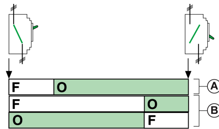
OF 触点与主触点关系的次序图
