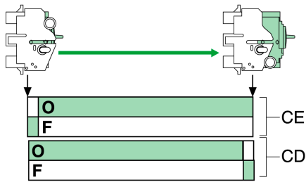
连接/退出位置触点的操作
