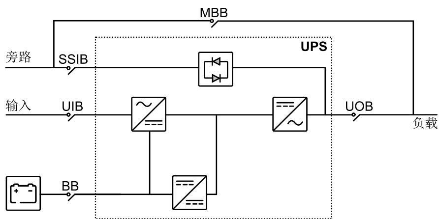
双市电系统
