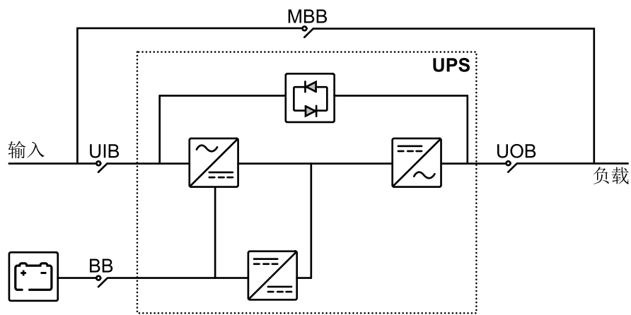
单市电系统
