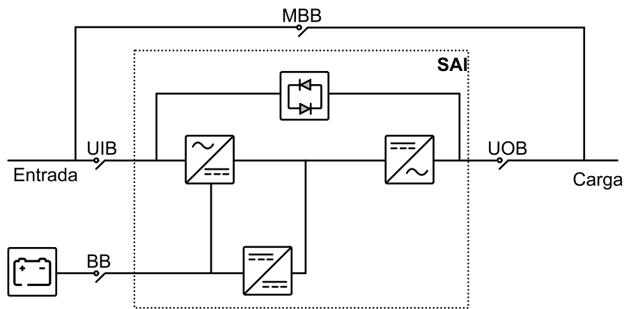
Sistema con suministro de red simple
