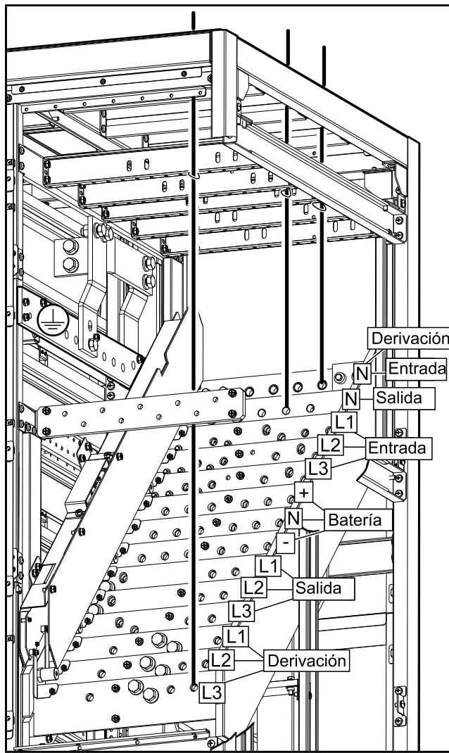
Sistema con suministro de red con dos entradas
