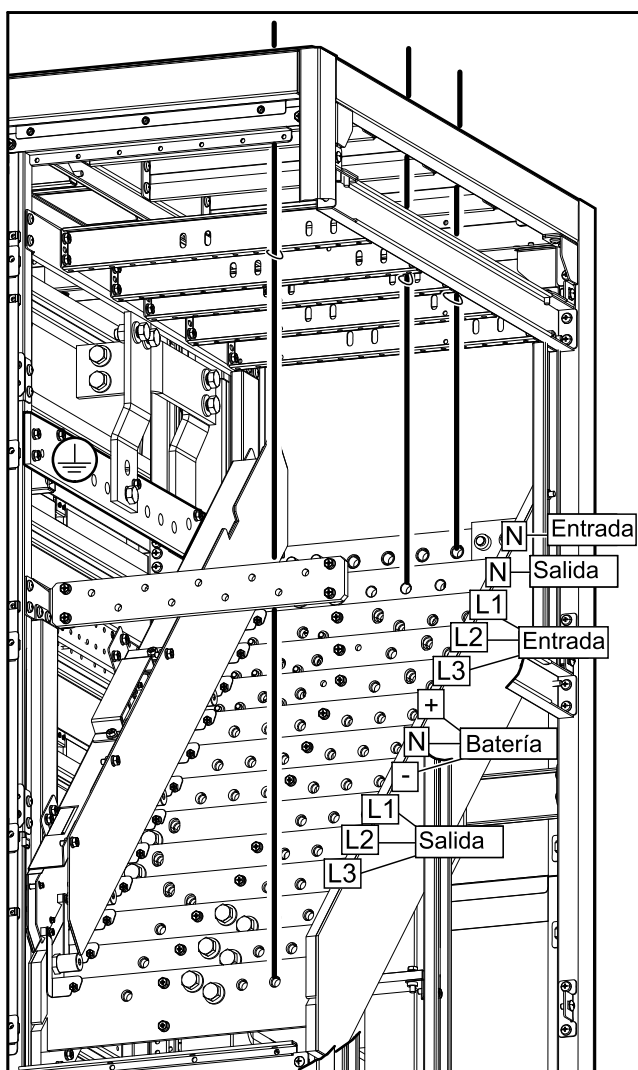
Sistema con suministro de red simple principal
