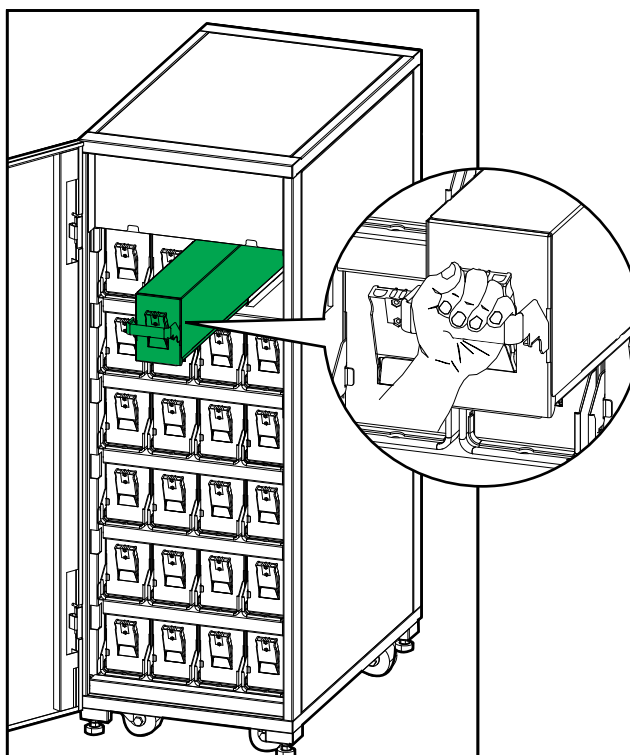
Vista anteriore dell'armadio delle batterie modulari
