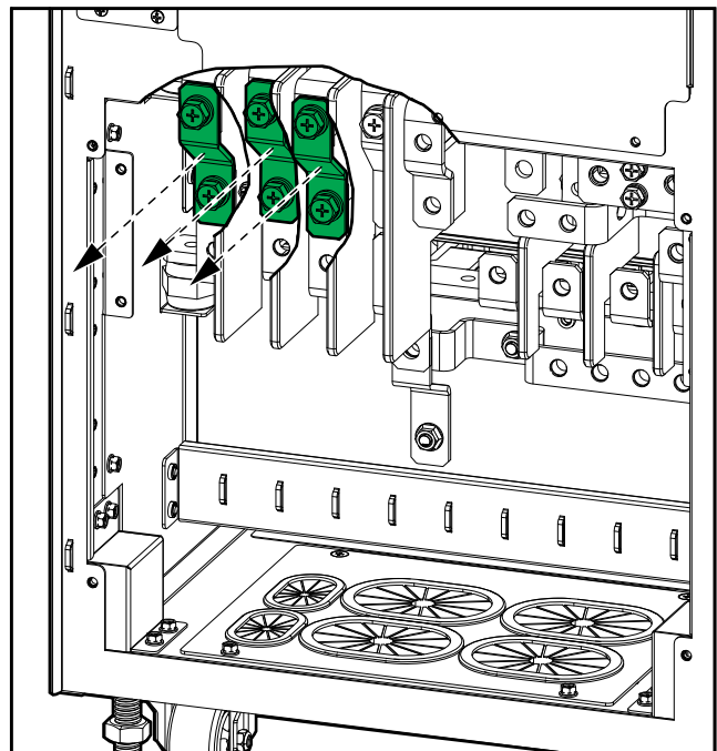
Vista posteriore 100 kVA 400 V/50 kVA 208 V UPS
