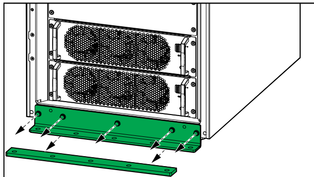
Vista frontal del SAI (con chapa de fijación)
