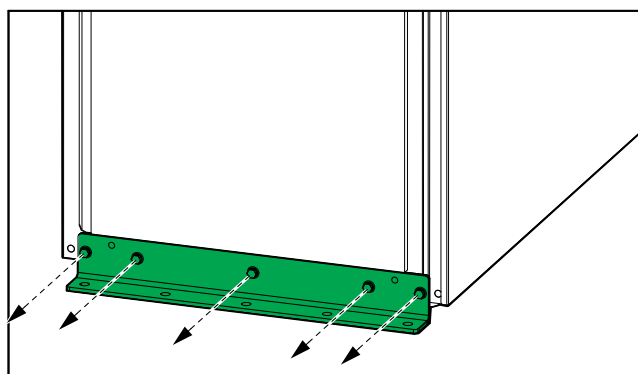
Vista trasera del SAI (sin chapa de fijación)
