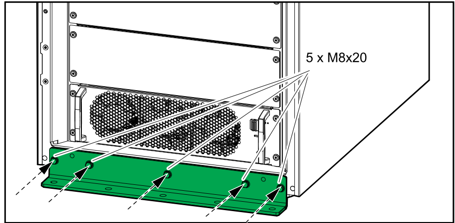
Vista frontal (con chapa de fijación)
