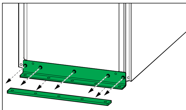
Vista trasera del SAI (con chapa de fijación)
