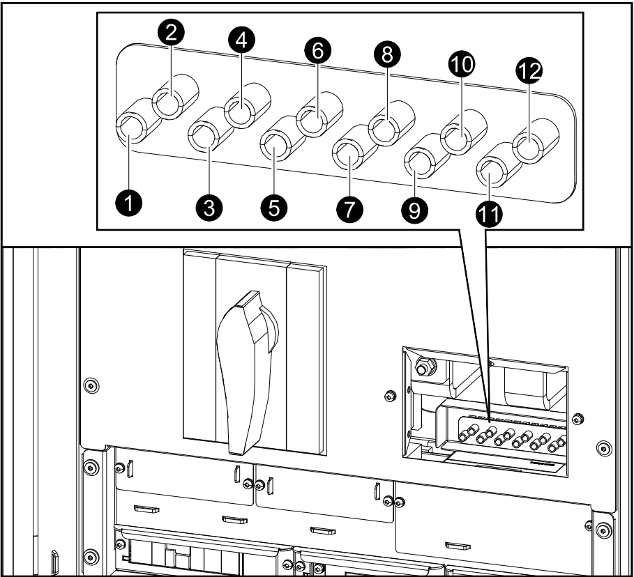
Vista frontal del SAI con un interruptor interno
