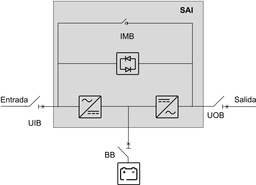
Sistema unitario – Suministro de red simple principal (un interruptor interno)
