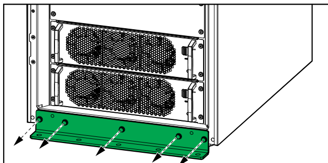
Widok zasilacza UPS z przodu (bez podkładki)
