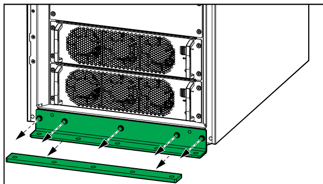
Widok zasilacza UPS z przodu (z podkładką)
