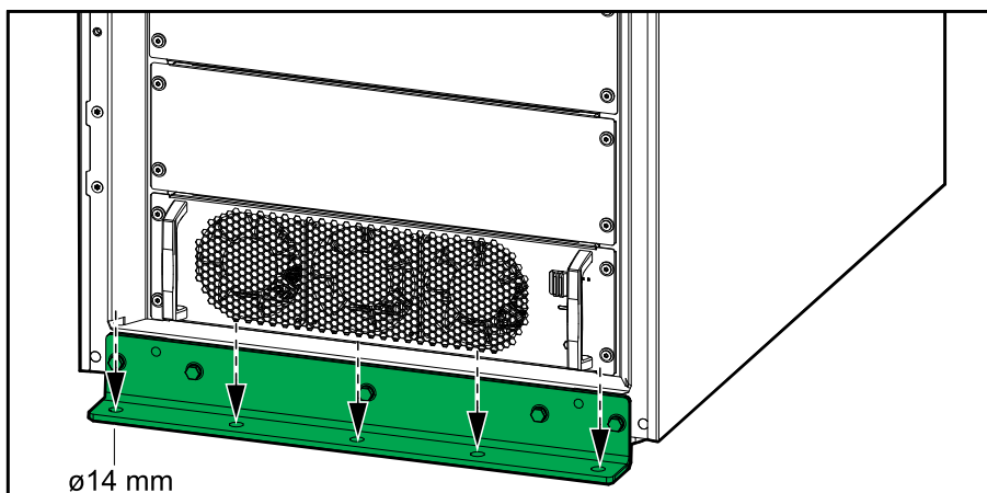
Widok z przodu (bez podkładki)
