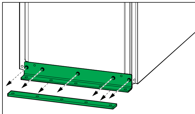
Widok zasilacza UPS z tyłu (z podkładką)
