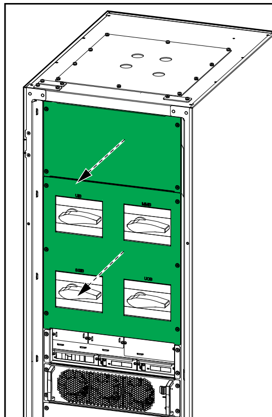
Zasilacz UPS z czterema wewnętrznymi przełącznikami
