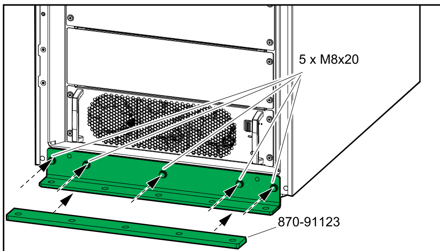
Widok z przodu (bez podkładki)
