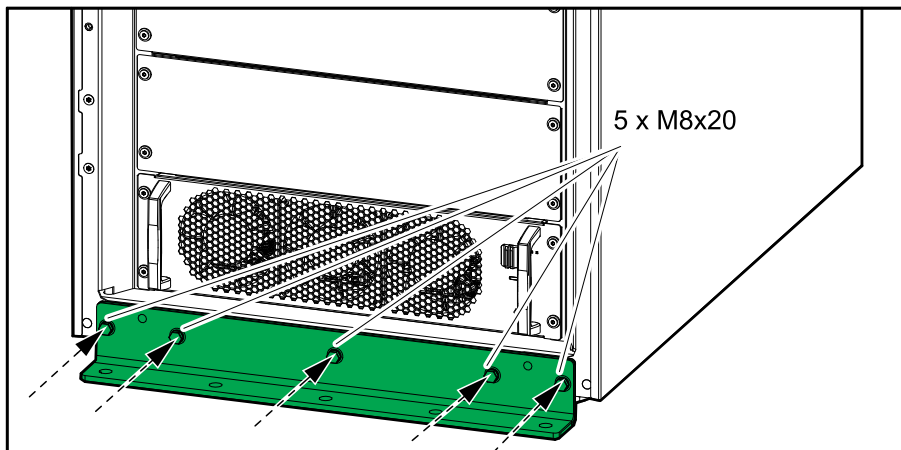
Widok z przodu (z podkładką)
