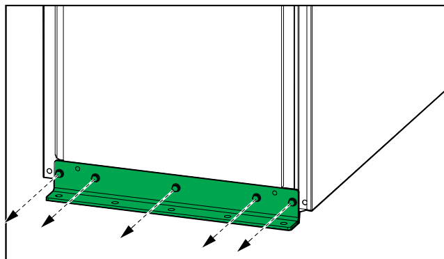
Widok zasilacza UPS z tyłu (bez podkładki)
