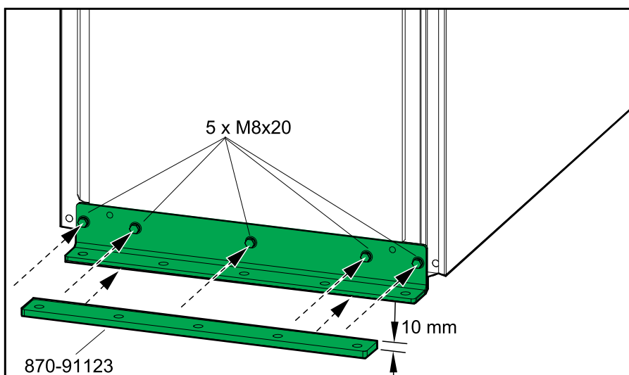
Widok z tyłu (z podkładką)
