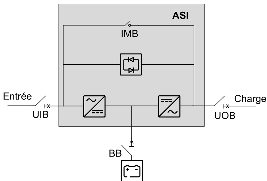
Système unitaire - Alimentation secteur simple (version onduleur avec 1 seul interrupteur)
