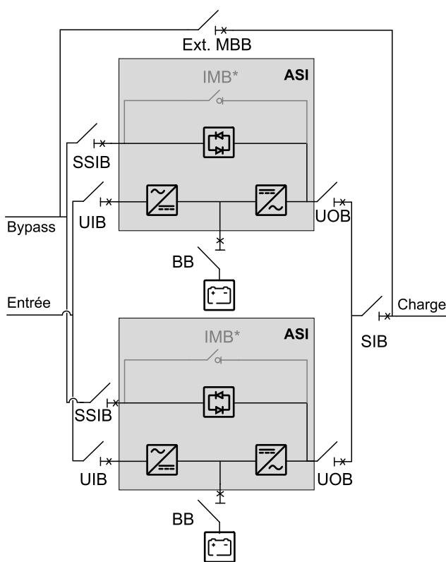
Système parallèle - Alimentation secteur double (un commutateur interne)
