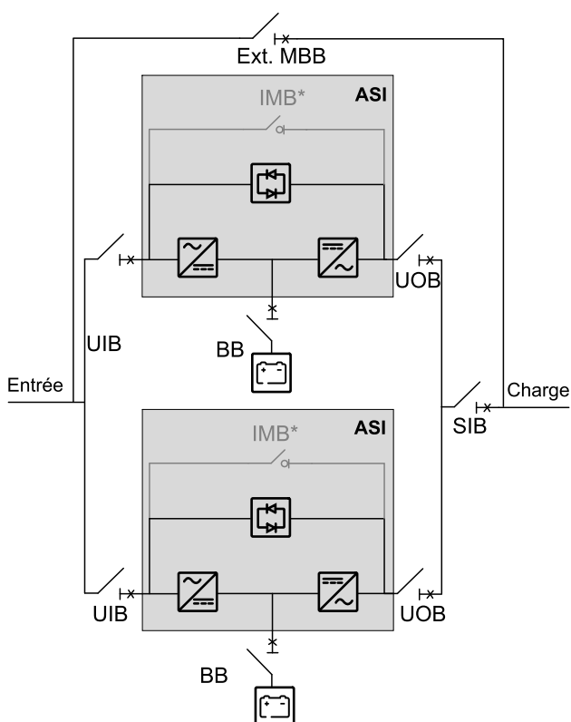
Système parallèle - Alimentation secteur simple (un commutateur interne)
