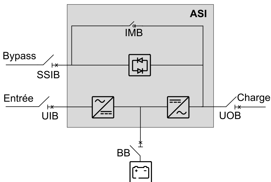
Système unitaire - Alimentation secteur double (version onduleur avec 1 seul interrupteur)
