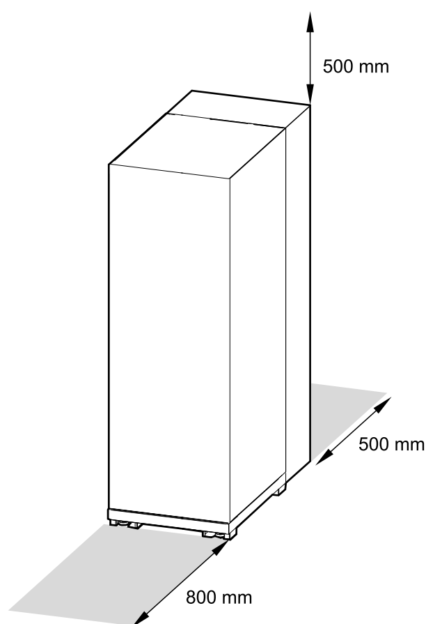
ASI avec adaptateur de profondeur
