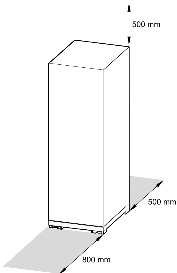
Zasilacz UPS
