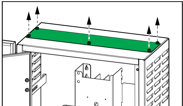
Vue supérieure de la partie avant du coffret disjoncteur batterie
