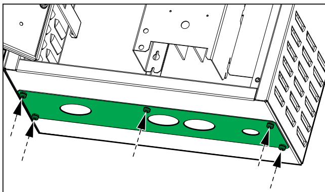
Vue inférieure de la partie avant du coffret disjoncteur batterie
