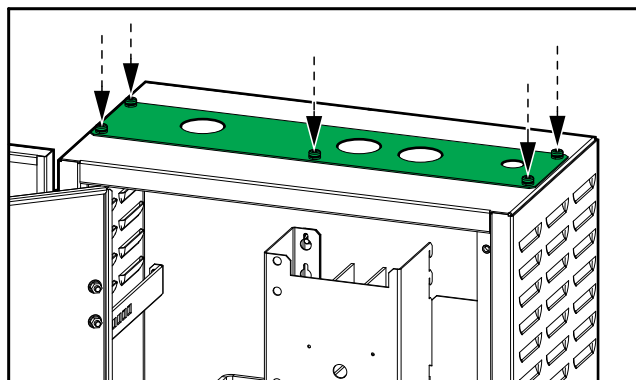
Vue supérieure de la partie avant du coffret disjoncteur batterie
