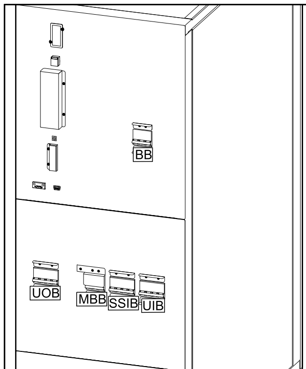
40 kVA 带内部电池的 UPS 背面视图
