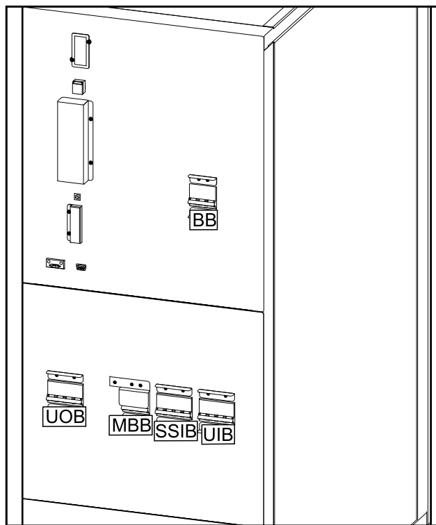
30 kVA 带内部电池的 UPS 背面视图
