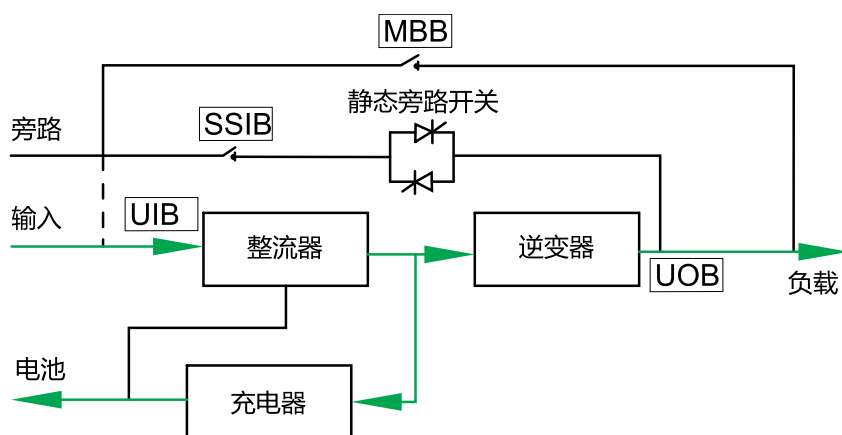
电流流向
