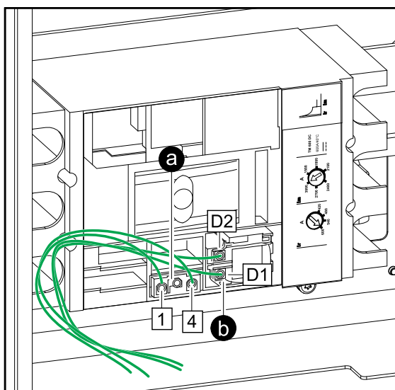
电池断路器正面视图
