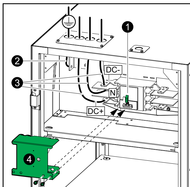
空电池柜正面视图 - 顶部线缆接入
