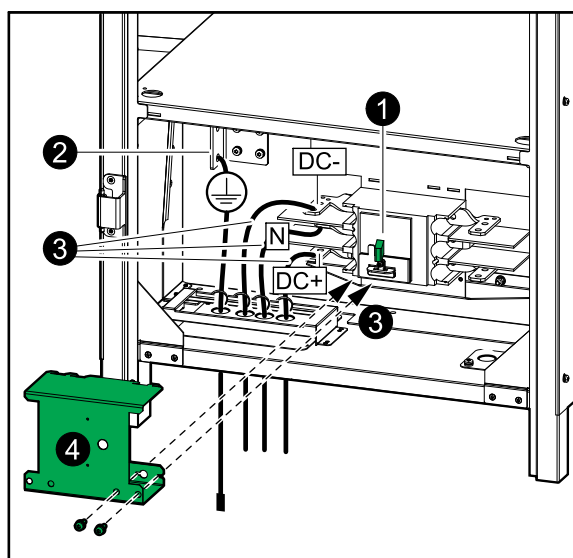
空电池柜正面视图 - 底部线缆接入
