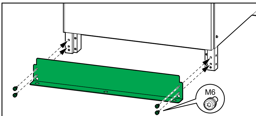
Vista frontal do gabinete de baterias vazio
