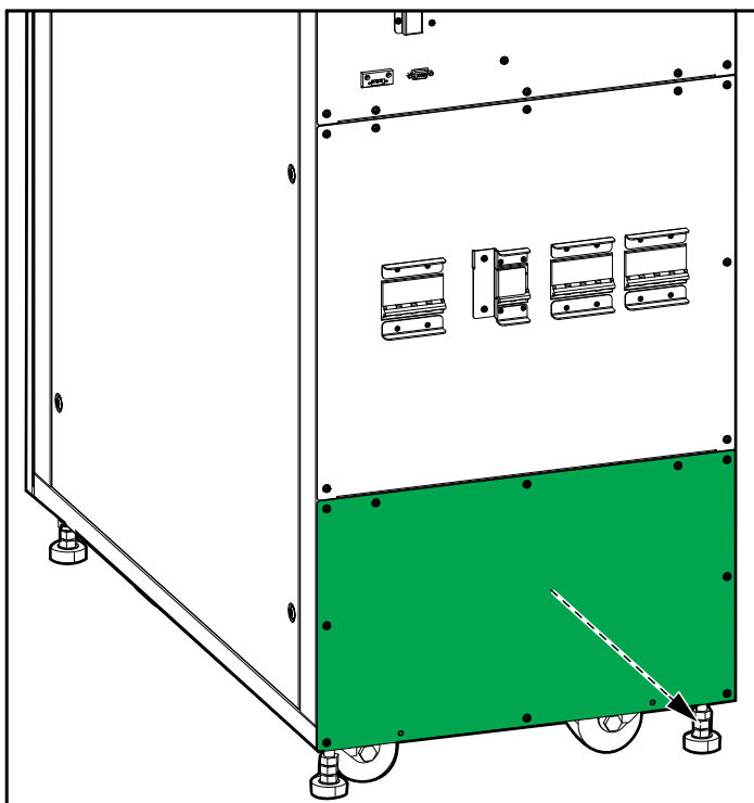
Vista posteriore dell'UPS da 30 kVA
