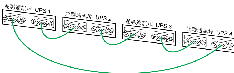
並聯板的頂部視圖
