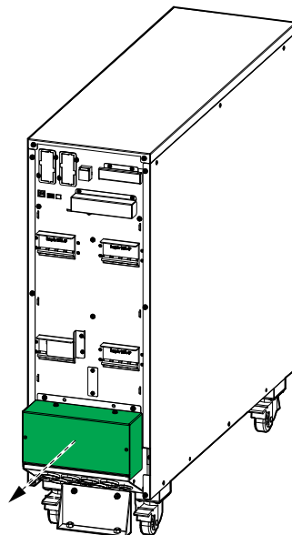
30-40 kVA UPS 的背部視圖
