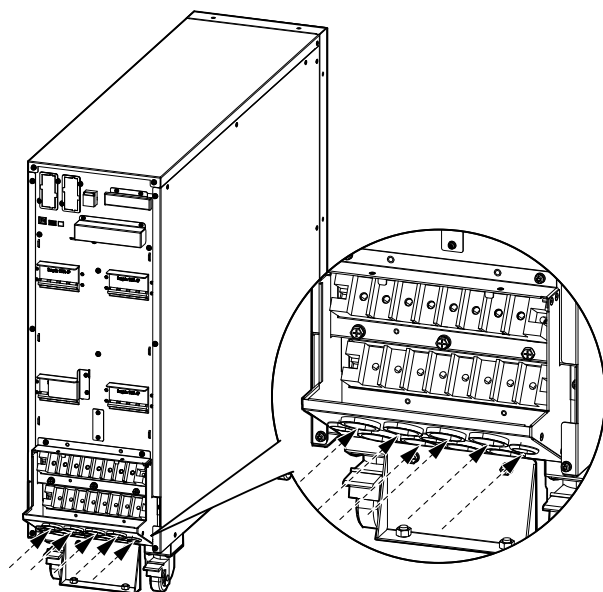
40 kVA UPS 背部視圖
