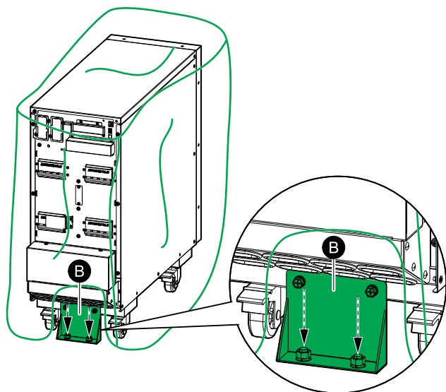
10-20 kVA UPS 的背部視圖
