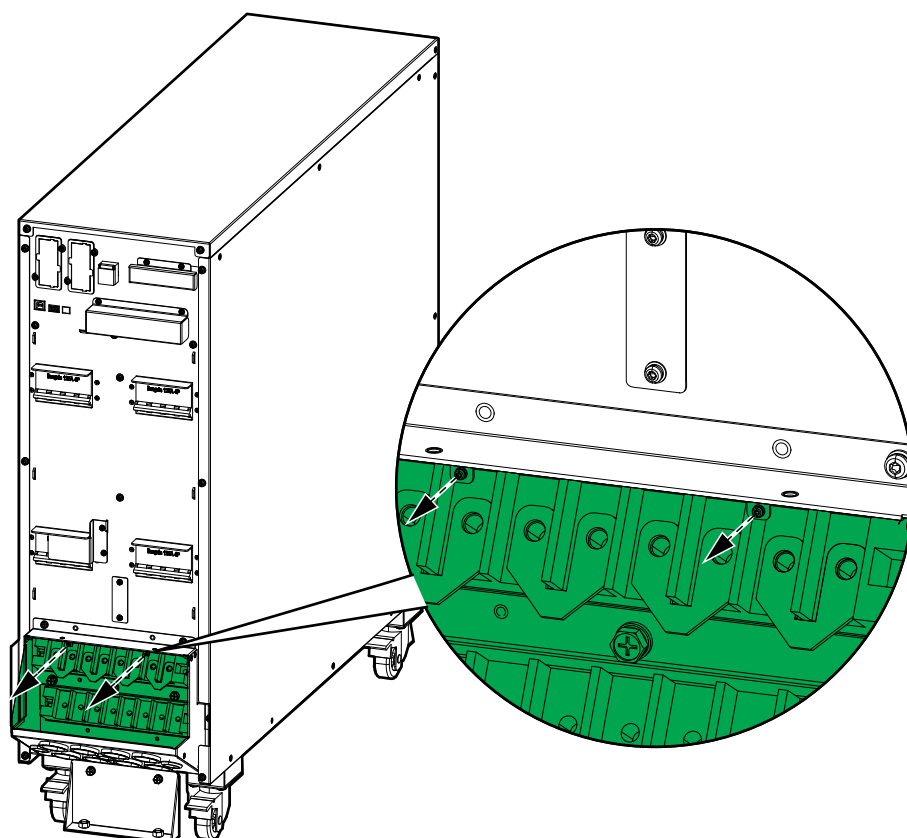
背部視圖
