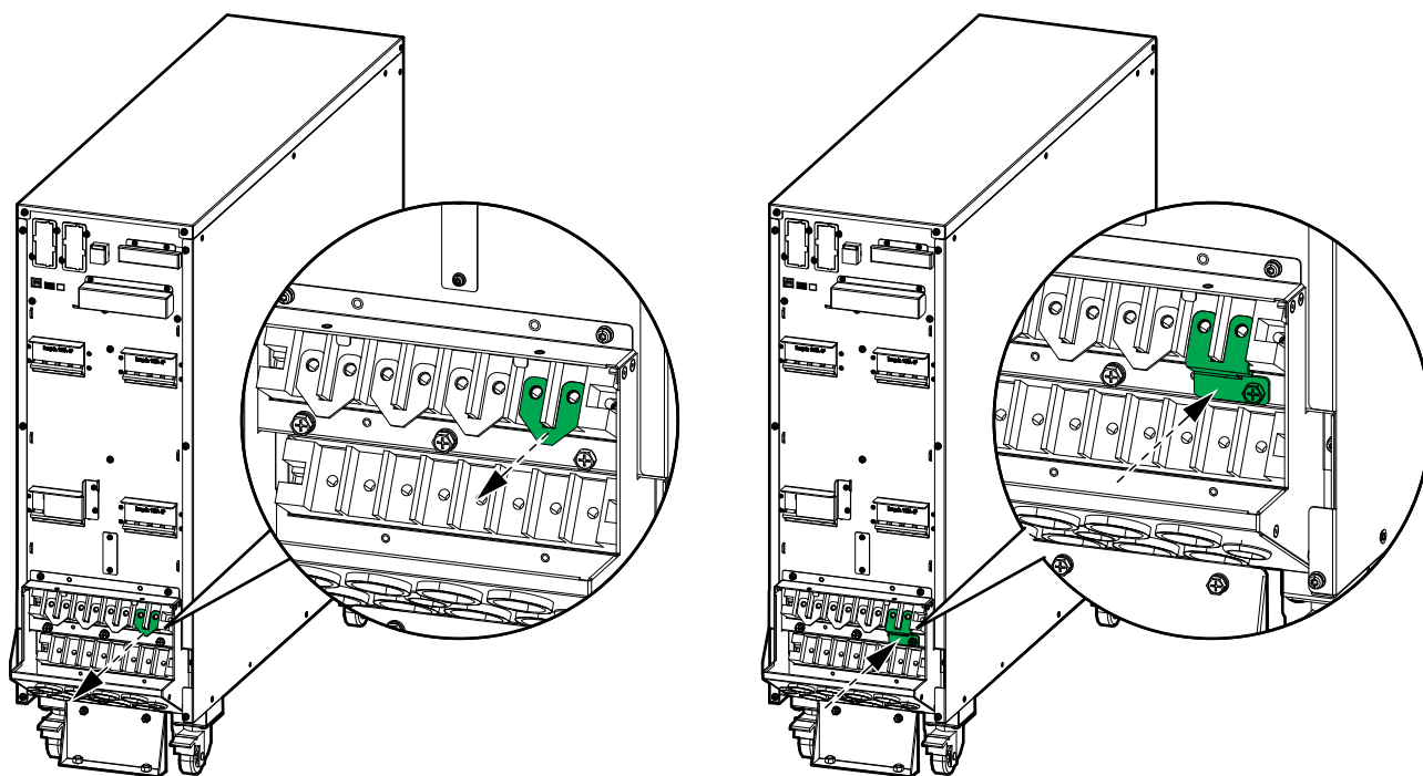
背部視圖 - TN-C 接地系統（單一主電源）
