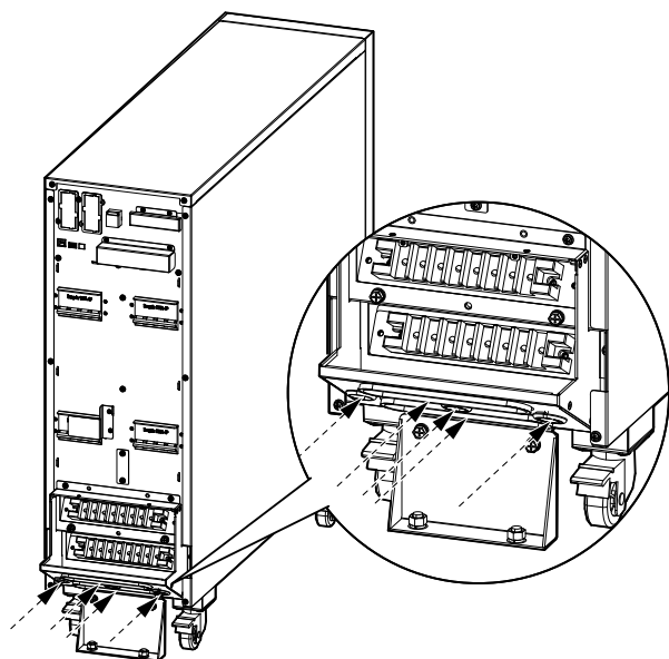
30 kVA UPS 背部視圖
