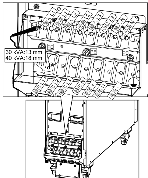
30-40 kVA UPS 的背部視圖
