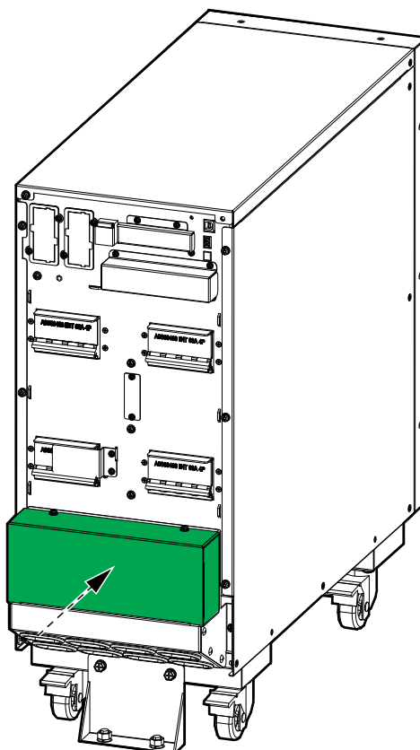
背部視圖
