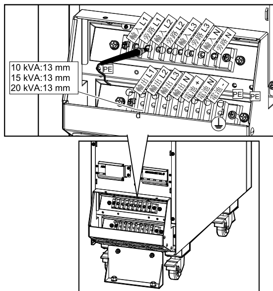
10-20 kVA UPS 的背部視圖
