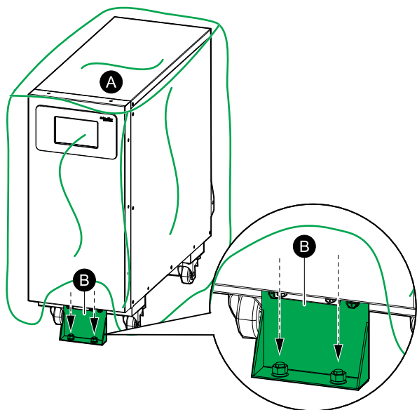
10-20 kVA UPS
