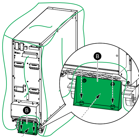
30-40 kVA UPS 的背部視圖
