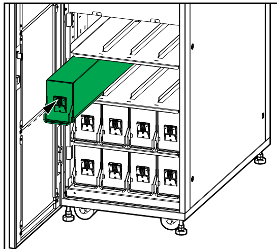
30–40 kVA UPS 正面视图
