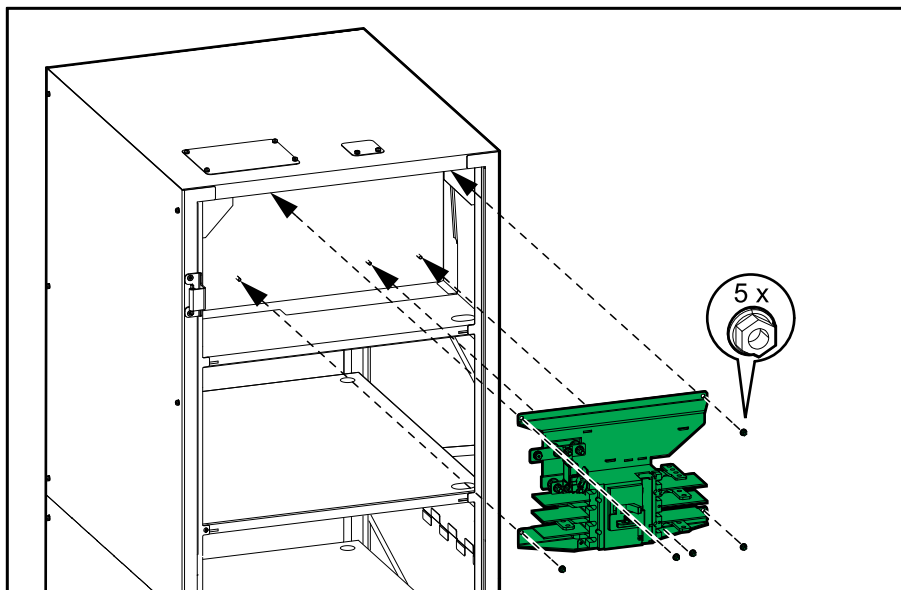
空电池柜正面视图
