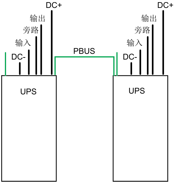
并机系统
