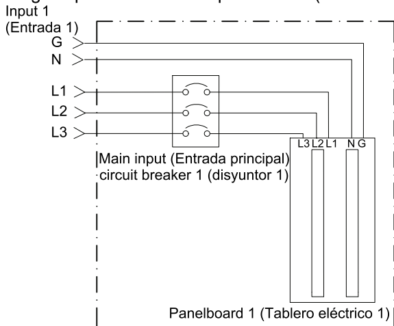
Single input source with 1 panelboard (Fuente de entrada simple con 1 tablero eléctrico)
