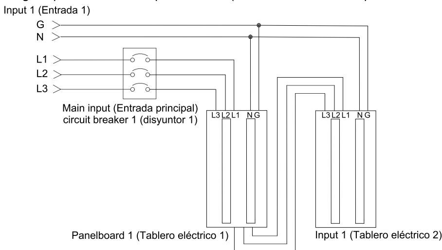
Single input source with 2 panelboards (Fuente de entrada simple con 2 tableros eléctricos)
