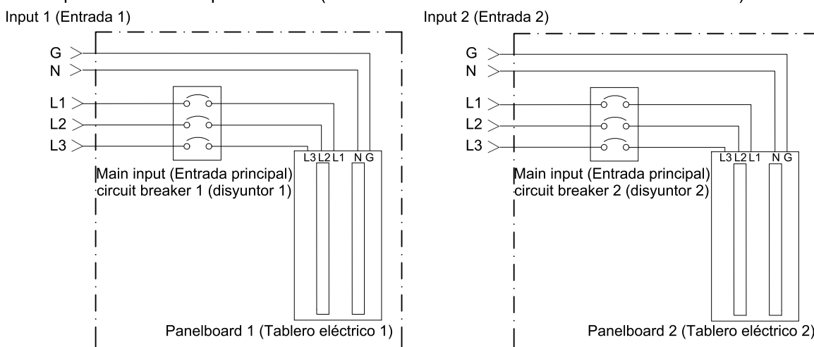
Dual input source with 2 panelboards (Fuente de entrada doble con 2 tableros eléctricos)
