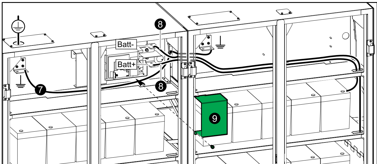
空のバッテリーキャビネット1と2の前面図
