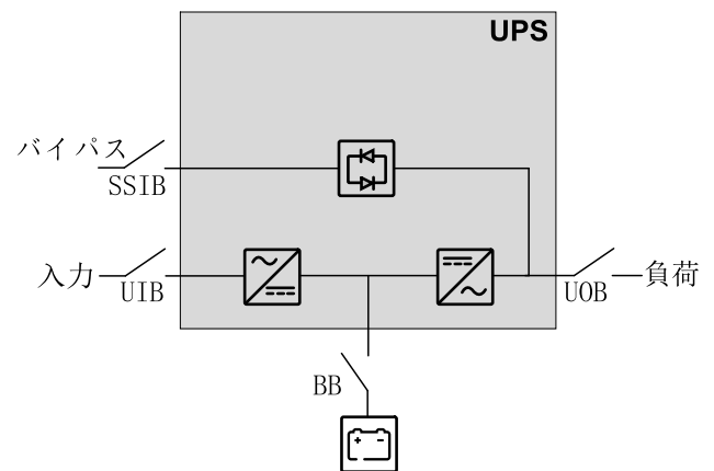
単機システム－デュアル給電
