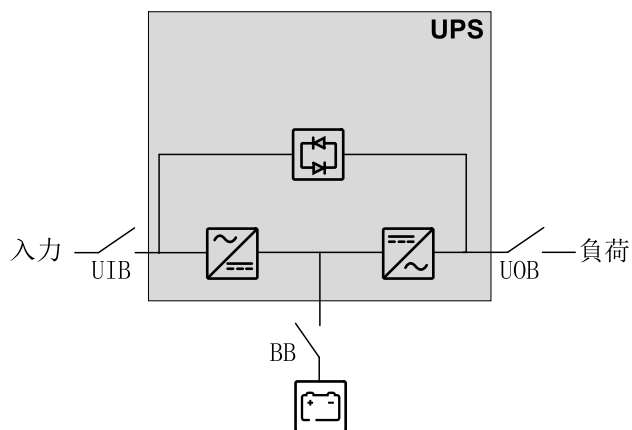
単機システム－シングル給電
