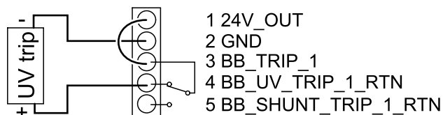
バッテリーブレーカートリップを24 VDC内部電源に接続する場合
