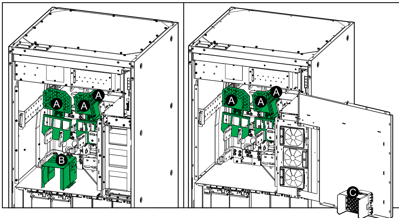
プラスチック製ボックスが分かれているUPSモデルの前面図 内側のドアにボックスを組み込んだUPSモデルの前面図
