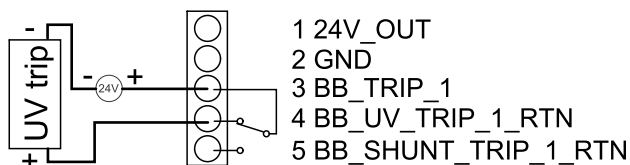
バッテリーブレーカートリップを24 VDC外部電源に接続する場合
