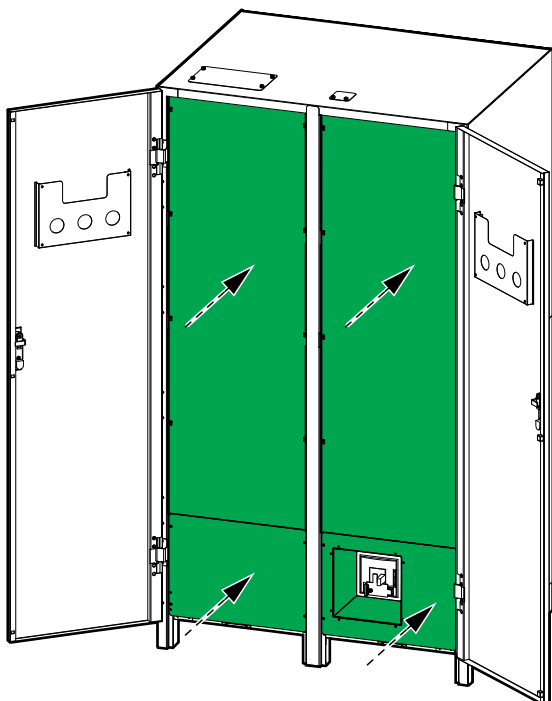
Σύστημα κάτω εισόδου καλωδίων
