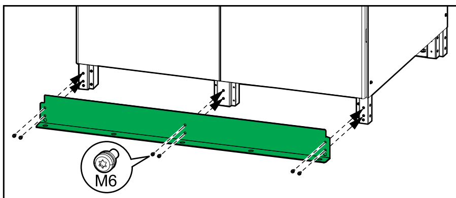
Vista frontal do gabinete de baterias vazio
