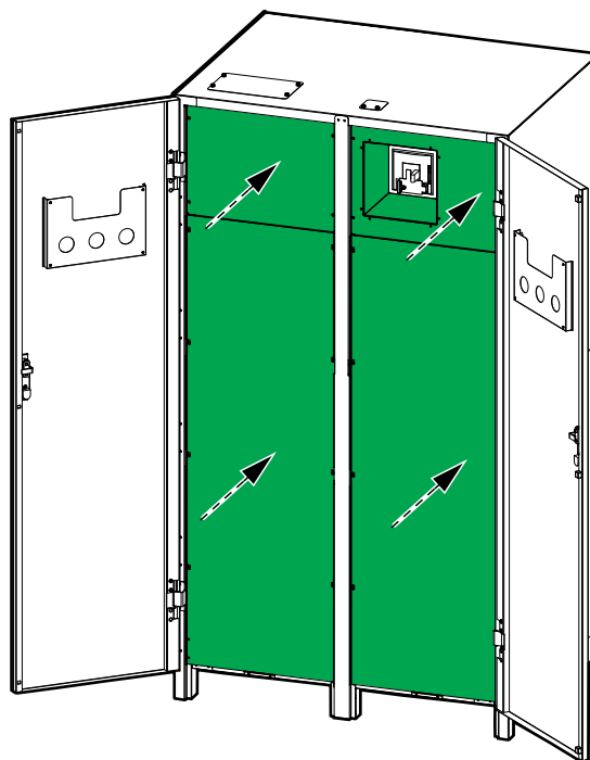
Sistema de entrada de cabos superior
