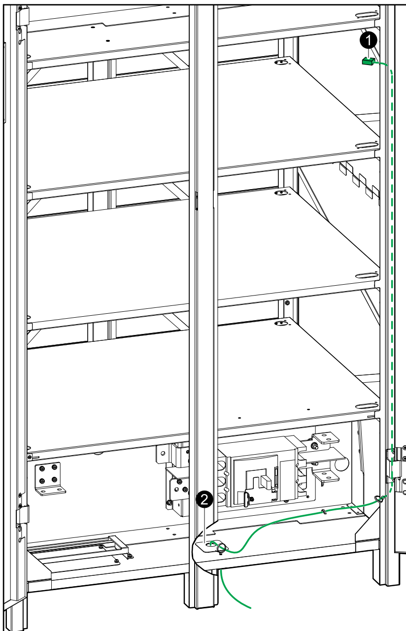
Widok z przodu pustej Szafy bateryjnej
