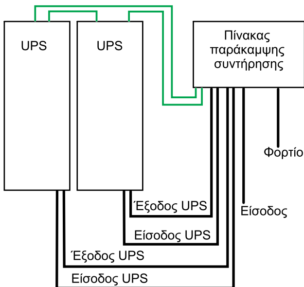
Απλοποιημένο παράλληλο σύστημα 1+1 – Ενιαία ηλεκτρική παροχή
