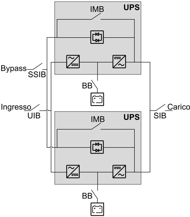
Sistema in parallelo 1 + 1 semplificato - Doppia rete di alimentazione
