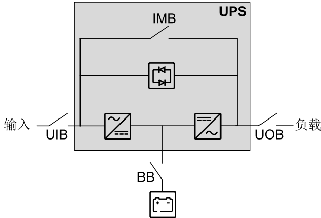
单机系统 - 单市电
