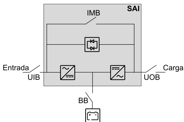
Sistema unitario: suministro de red simple
