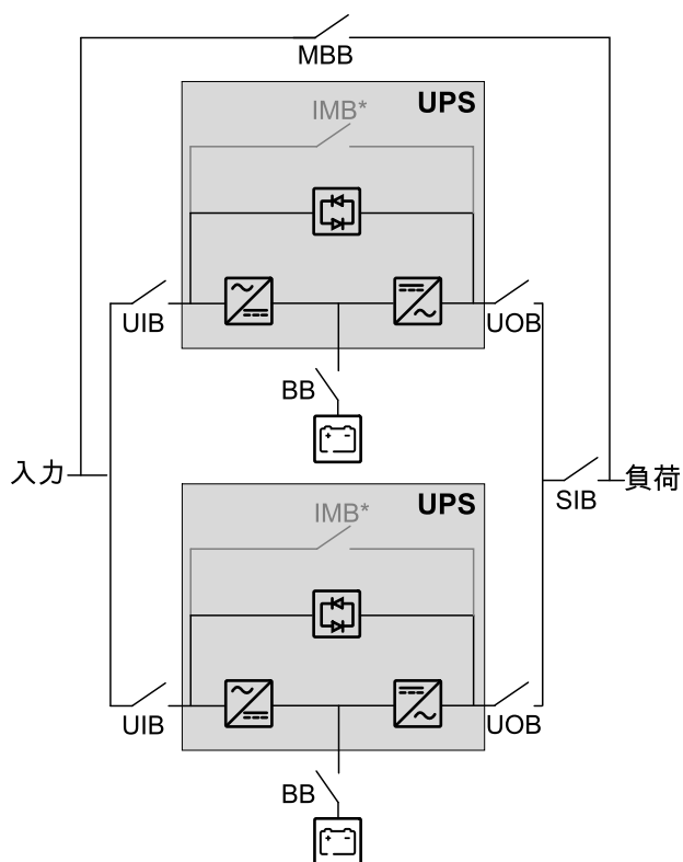
並列システム- 1系統主電源
