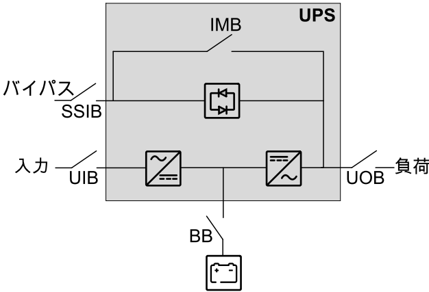
単機システム - 2系統主電源
