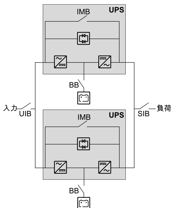
1+1簡易並列システム- 1系統主電源
