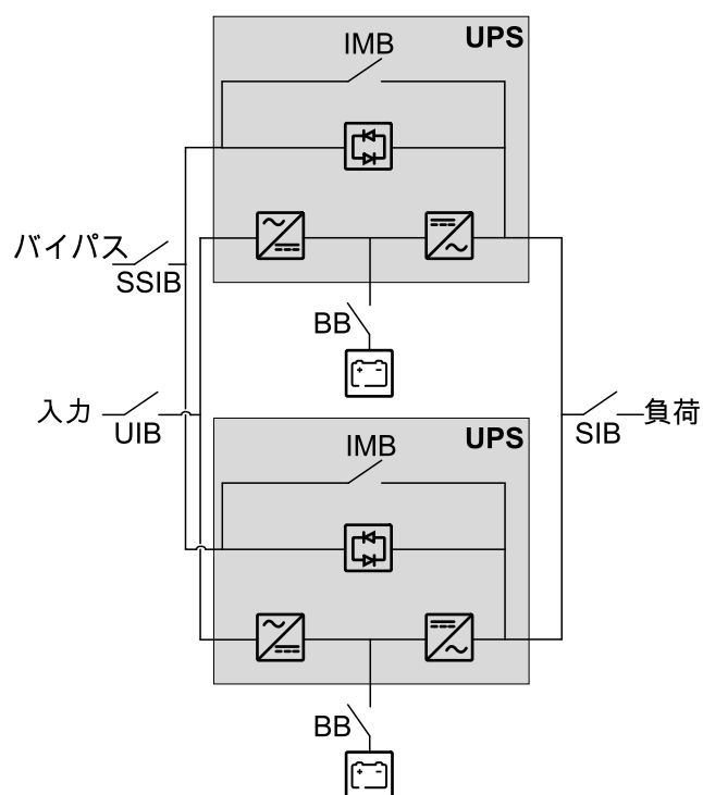
1+1簡易並列システム- 2系統主電源
