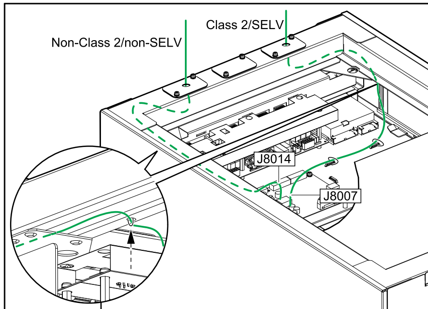
UPS 顶部视图
