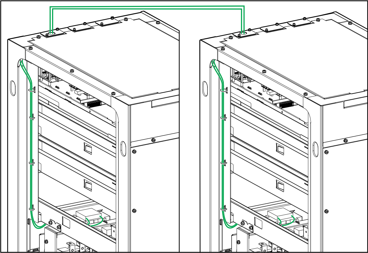
简化 1+1 并机系统背面右侧视图
