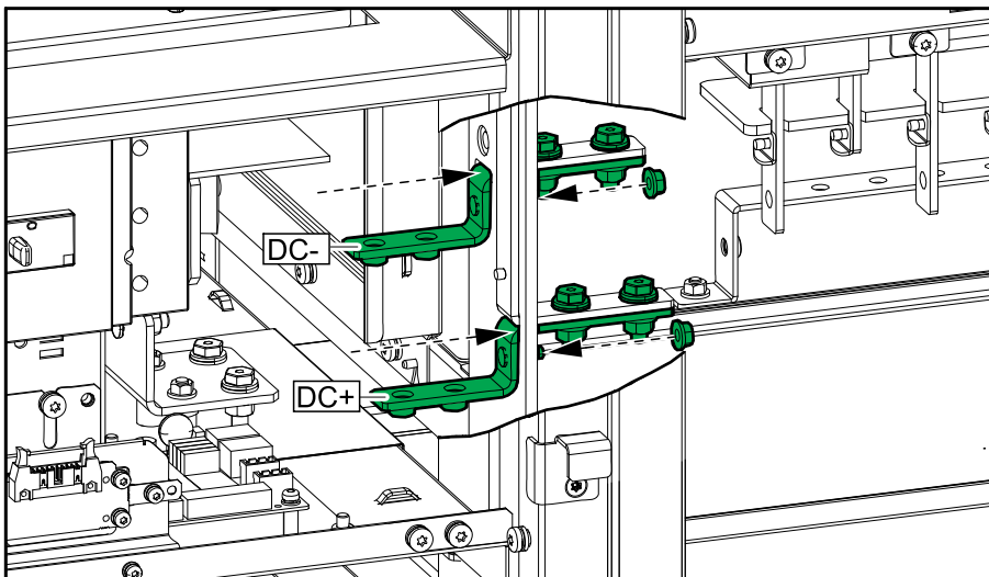
模块电池柜 1 和 UPS 的正面视图
