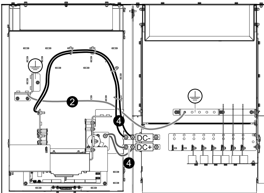
模块电池柜 1 和 UPS 的顶部视图
