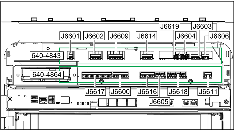
UPS 正面视图 - 电路板 640-4843 和 640-4864
