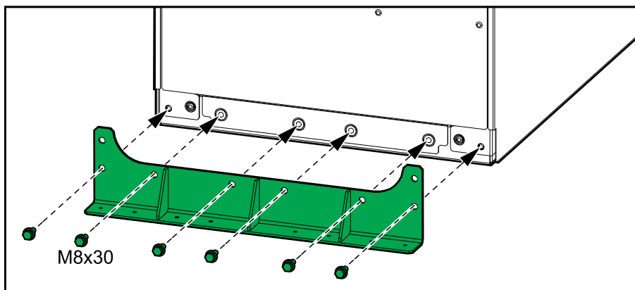
UPS 背面视图
