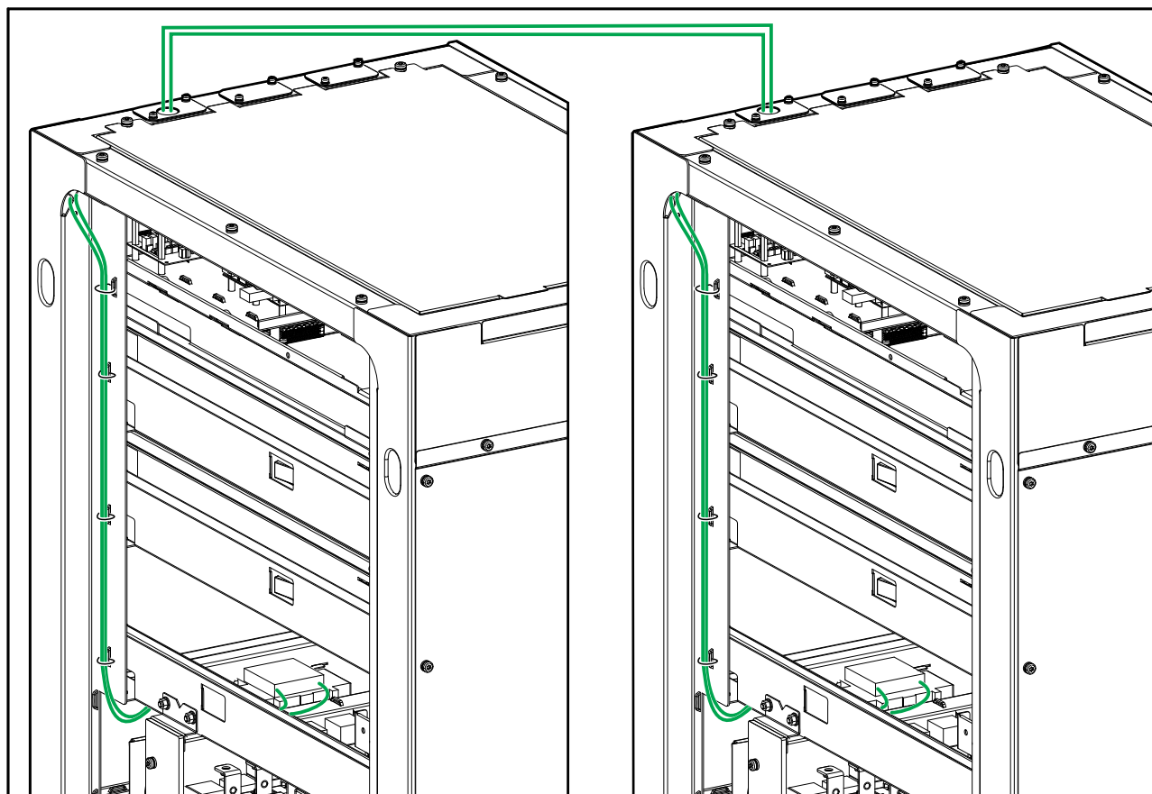
1+1簡易並列システムの背面右側面図
