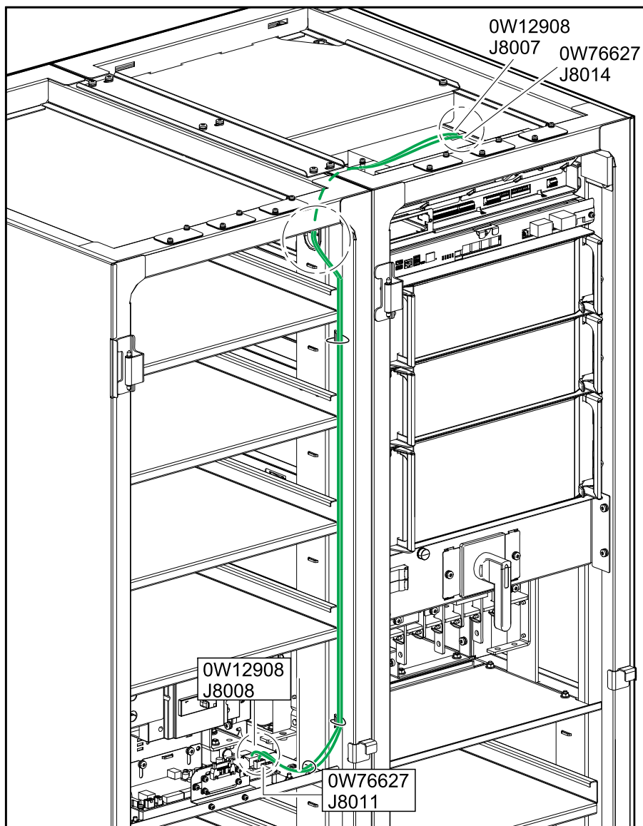
隣接するモジュール式バッテリーキャビネット1とUPSの前面図
