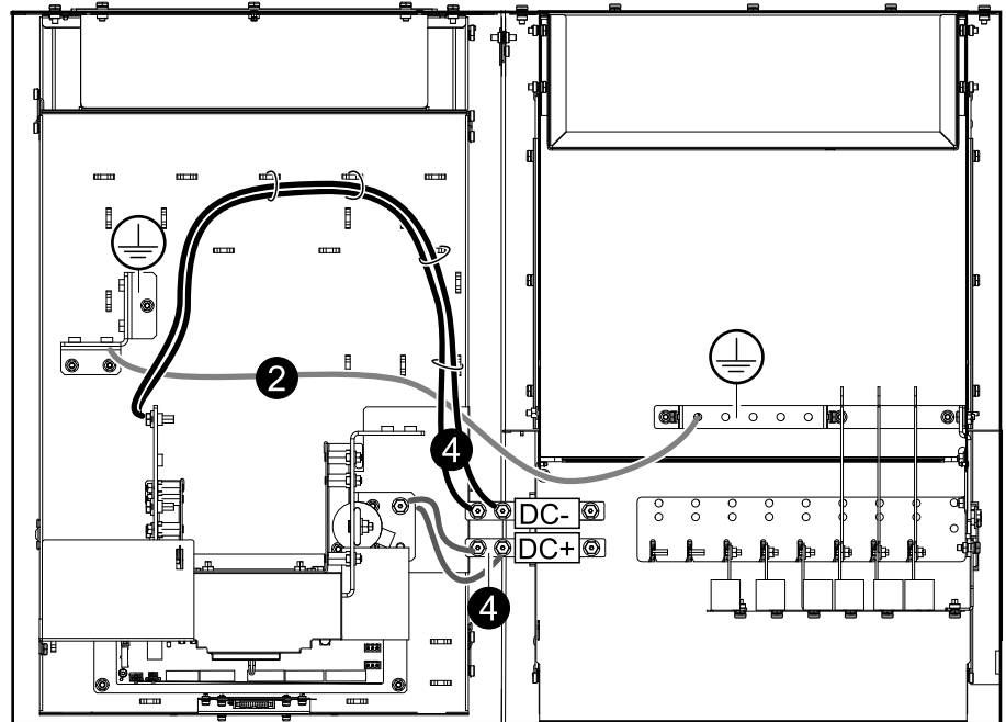
モジュール式バッテリーキャビネット1とUPSの上面図
