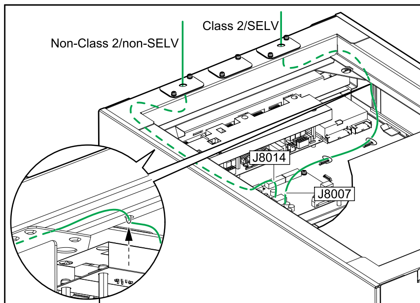
UPSの上面図
