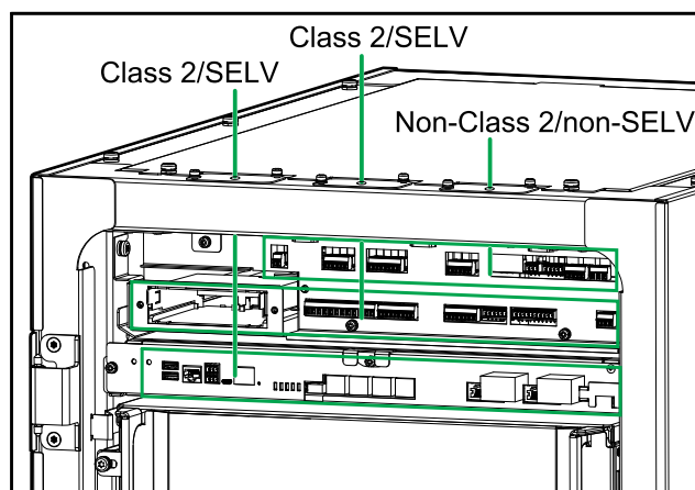
UPS med kabelkanaler
