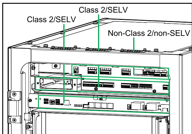
UPS ที่ไม่มีท่อร้อยสาย
