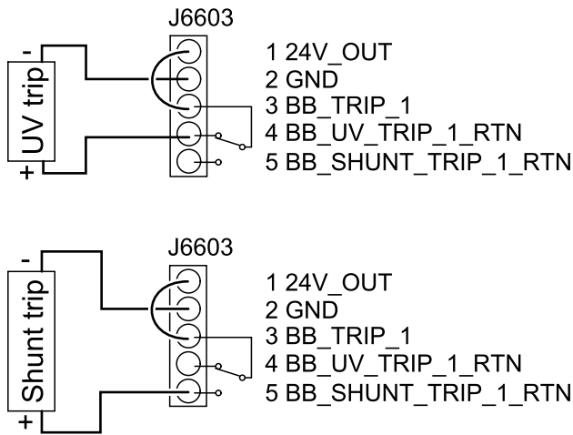
电池断路器脱扣与内部 24 VDC 电源连接
