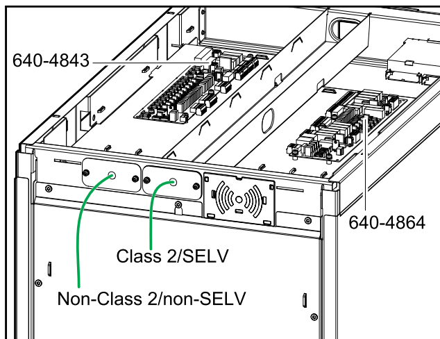
UPS 背面视图（带导线管）
