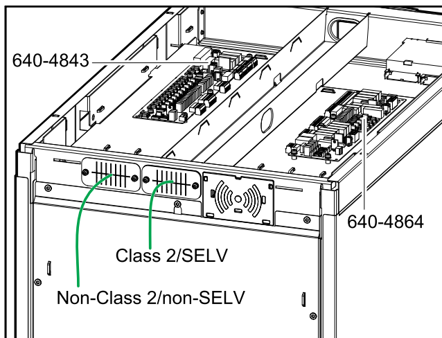
UPS 背面视图（不带导线管）
