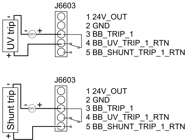
电池断路器脱扣与外部 24 VDC 电源连接
