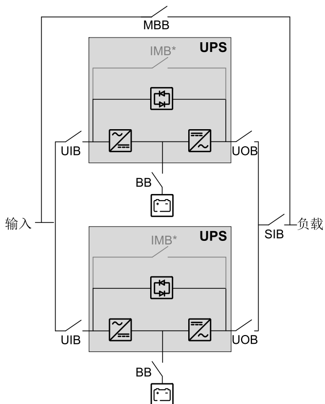
并机系统- 单市电
