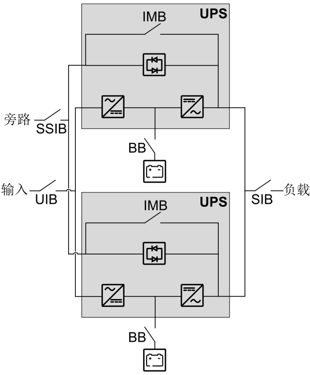
简化1+1 并机系统- 双市电
