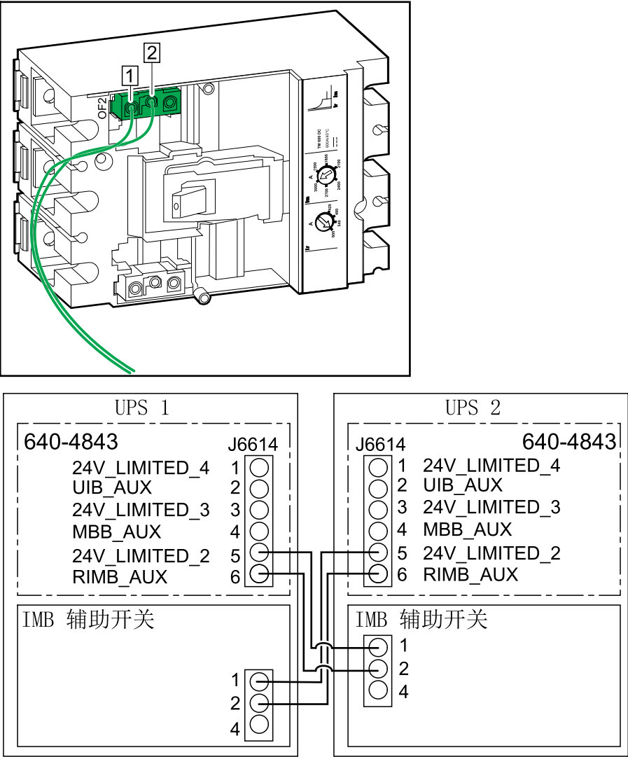
内部维修断路器 (IMB) 正面视图
