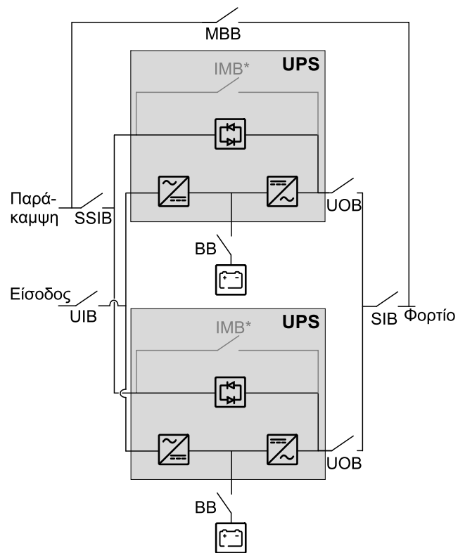
Παράλληλο σύστημα – Διπλή ηλεκτρική παροχή
