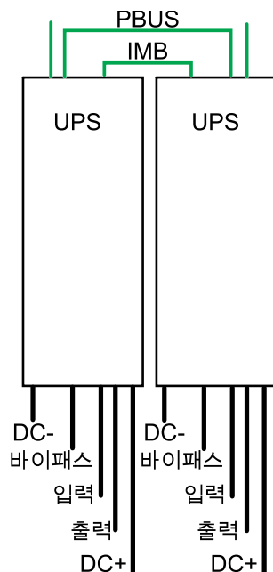
단순화된 1+1 병렬 시스템
