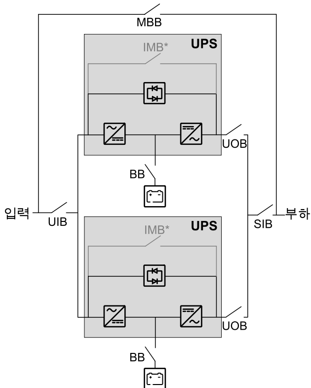
병렬 시스템 - 단독 주 전원
