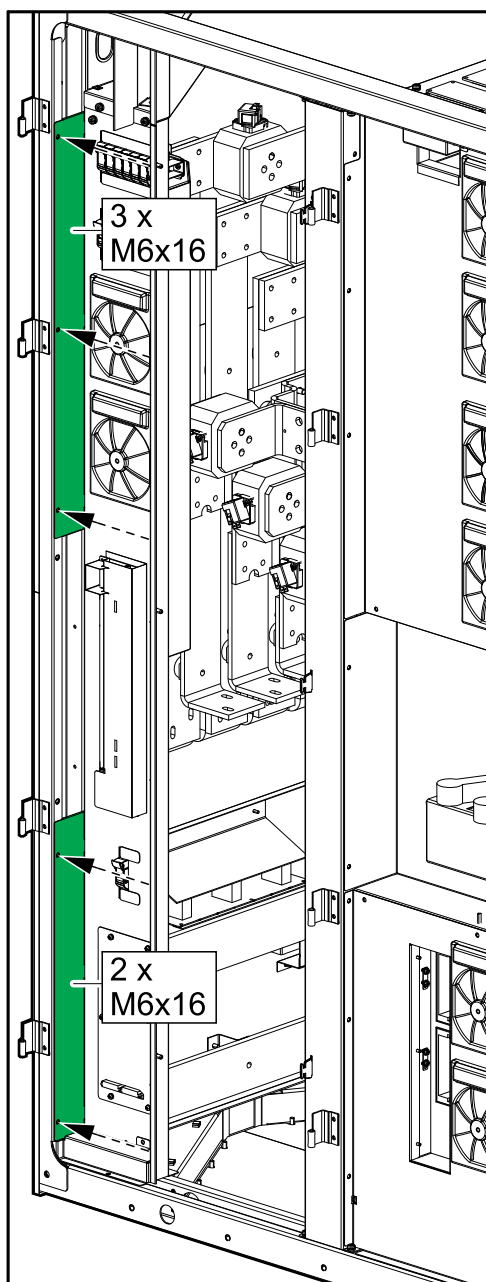
I/O 机柜正面视图
