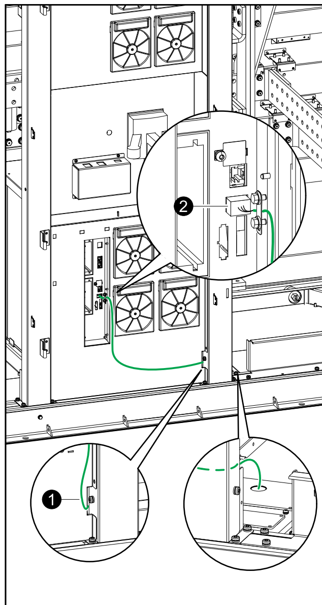
底部进线系统的 I/O 机柜正面视图
