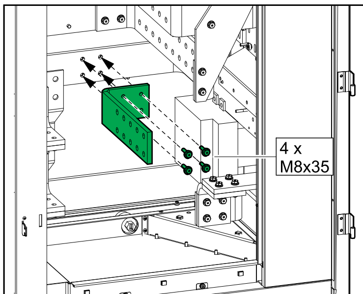
I/O 机柜正面视图
