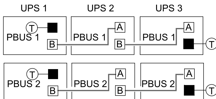
Eksempel på system med tre UPS'er i parallel
