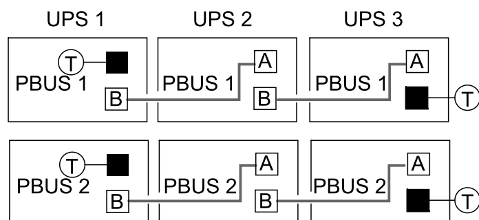
3台のUPSを並列に接続したシステムの例
