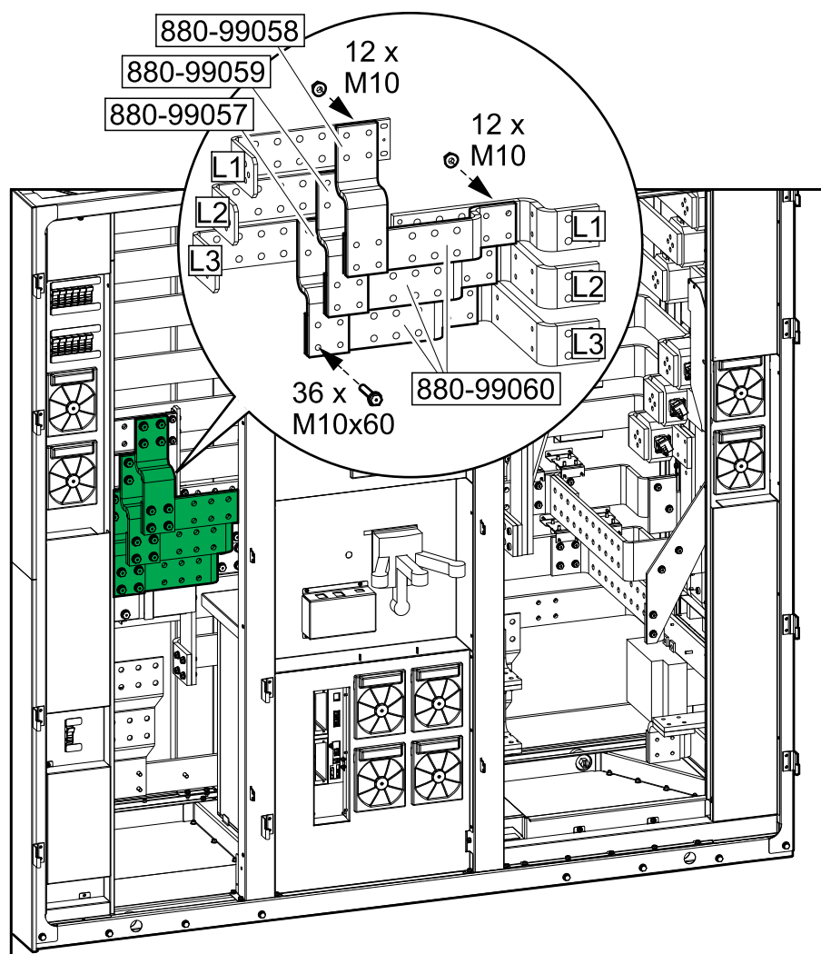
I/Oキャビネットの前面図
