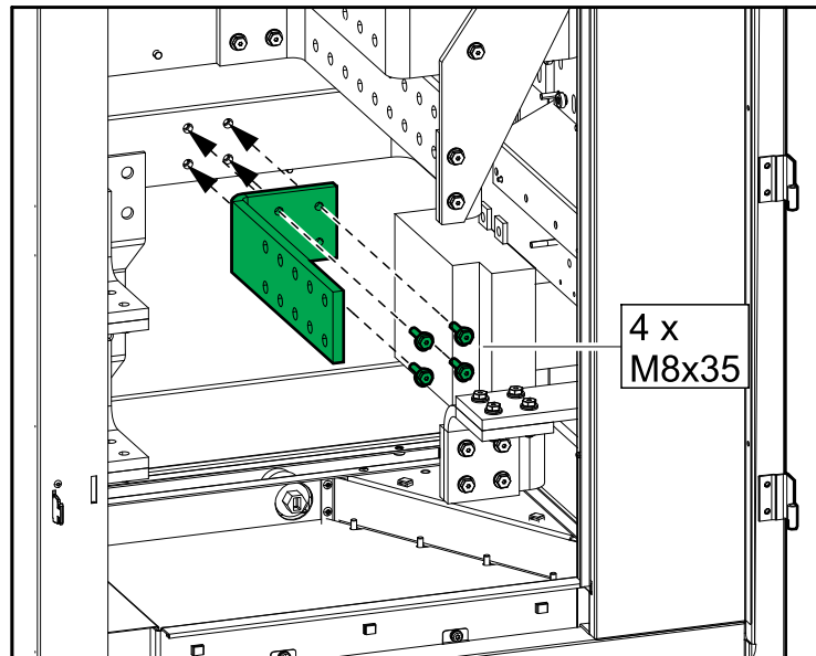
I/Oキャビネットの前面図
