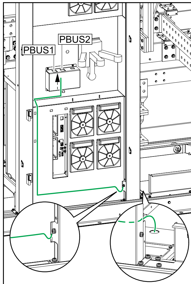
下部入線システムの場合
