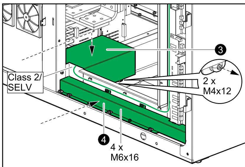
I/Oキャビネットの前面図
