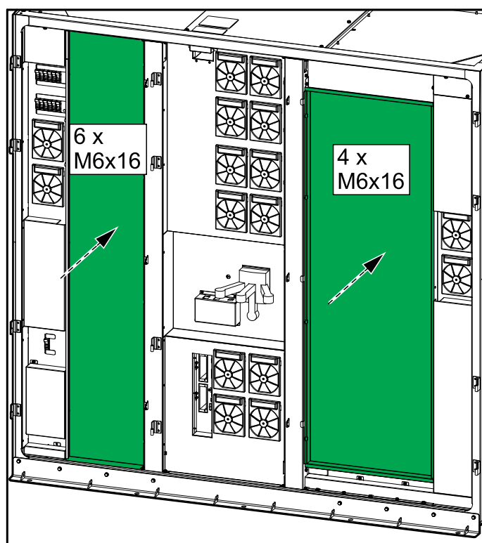
I/Oキャビネットの前面図
