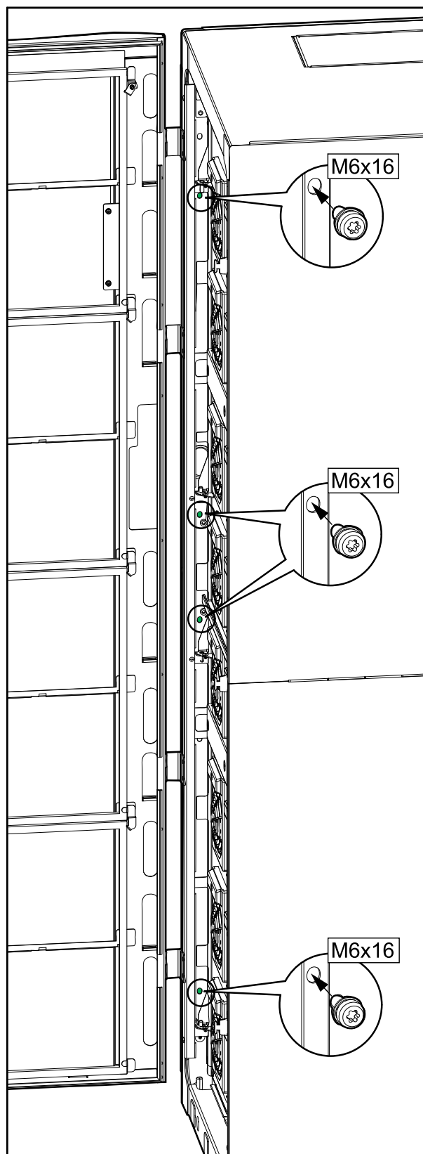
I/Oキャビネットの右側にあるパワーキャビネットをI/Oキャビネットに固定
