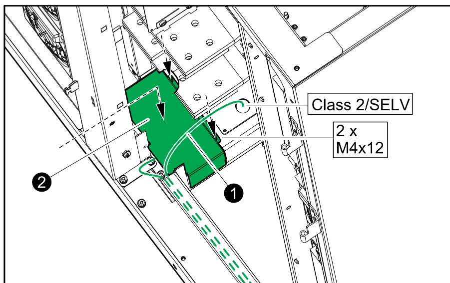
I/Oキャビネットの前面図
