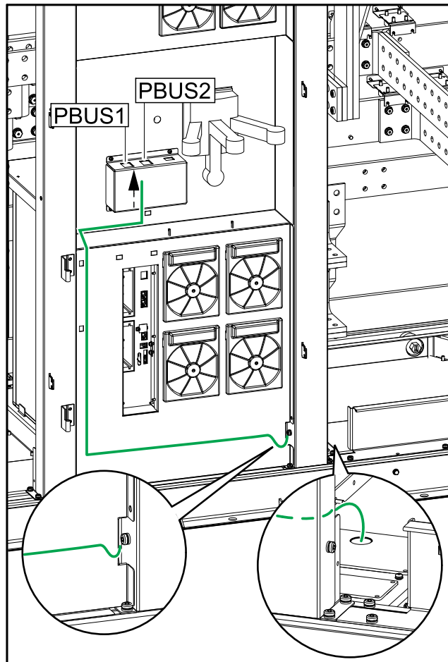
Sistemas con entrada de cables por la parte inferior
