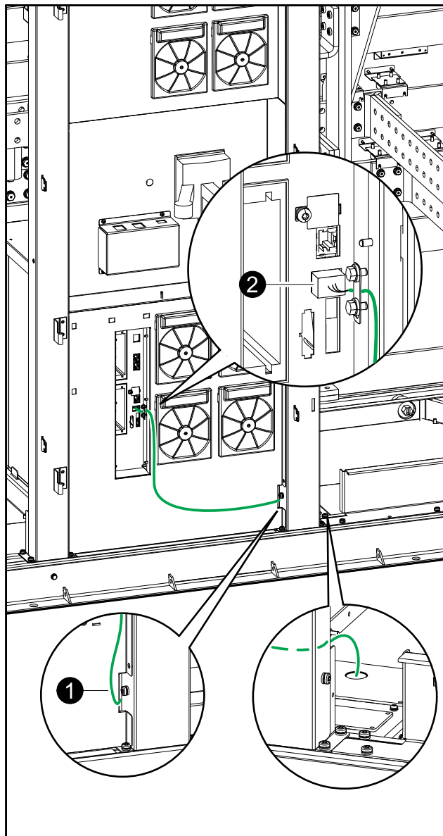
Vista frontal del armario de E/S en sistemas con entrada de cables por la parte inferior
