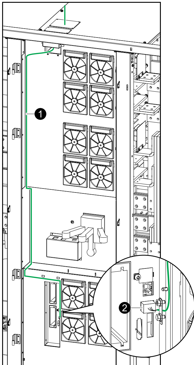
Vista frontal del armario de E/S en sistemas con entrada de cables por la parte superior
