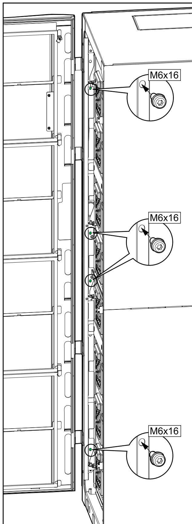
パワーキャビネットとI/Oキャビネット間のネジ位置
