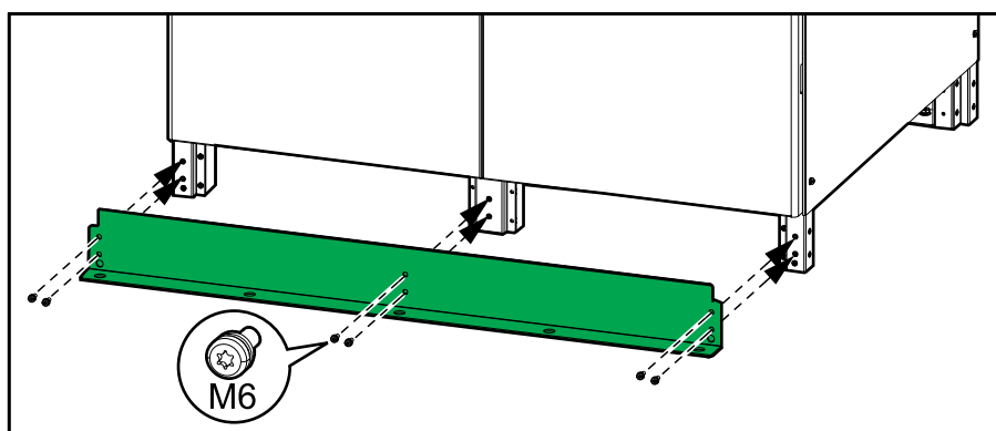
Tomt batterikabinett vist forfra
