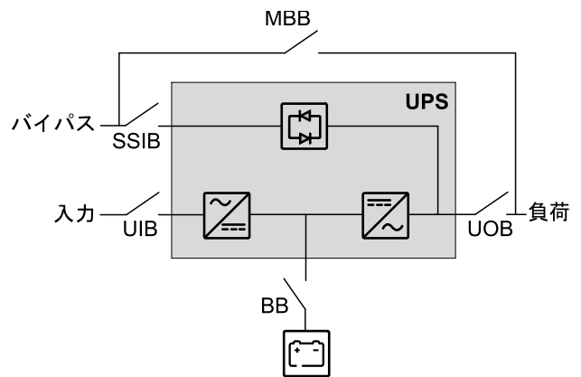
単機システム - 2系統主電源
