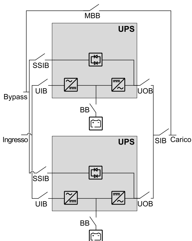
Sistema in parallelo - Alimentazione doppia
