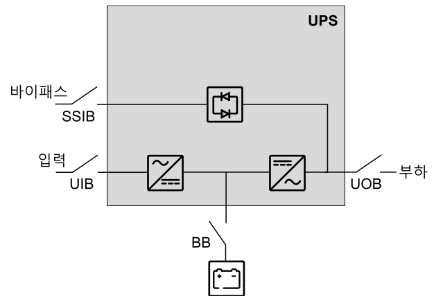
단일 시스템 - 이중 입력 전원
