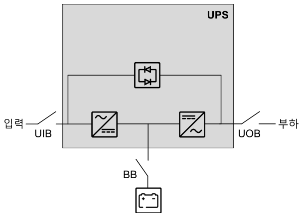
단일 시스템 - 단일 입력 전원
