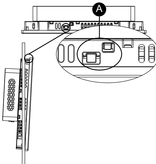
A. Fallsicherung
