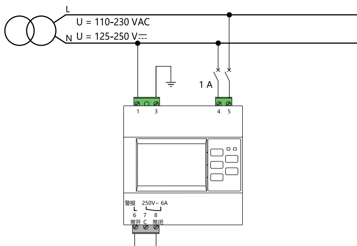
IM15H / IM20-H 接线图：
